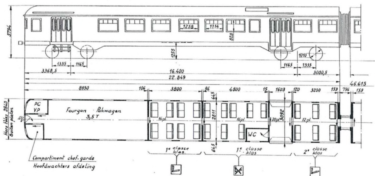
Voiture AB à partir de 1979 (Recueil des schémas des automotrices de la SNCB. 1935-1986, J. Vandenberghe, 1987, p. 62.)
