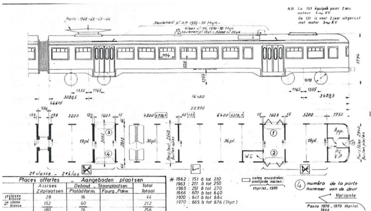
Schema van een B-rijtuig (Verzameling schema's van de motorrijtuigen van de NMBS. 1935-1986, J. Vandenberghen, 1987, p. 56.)
