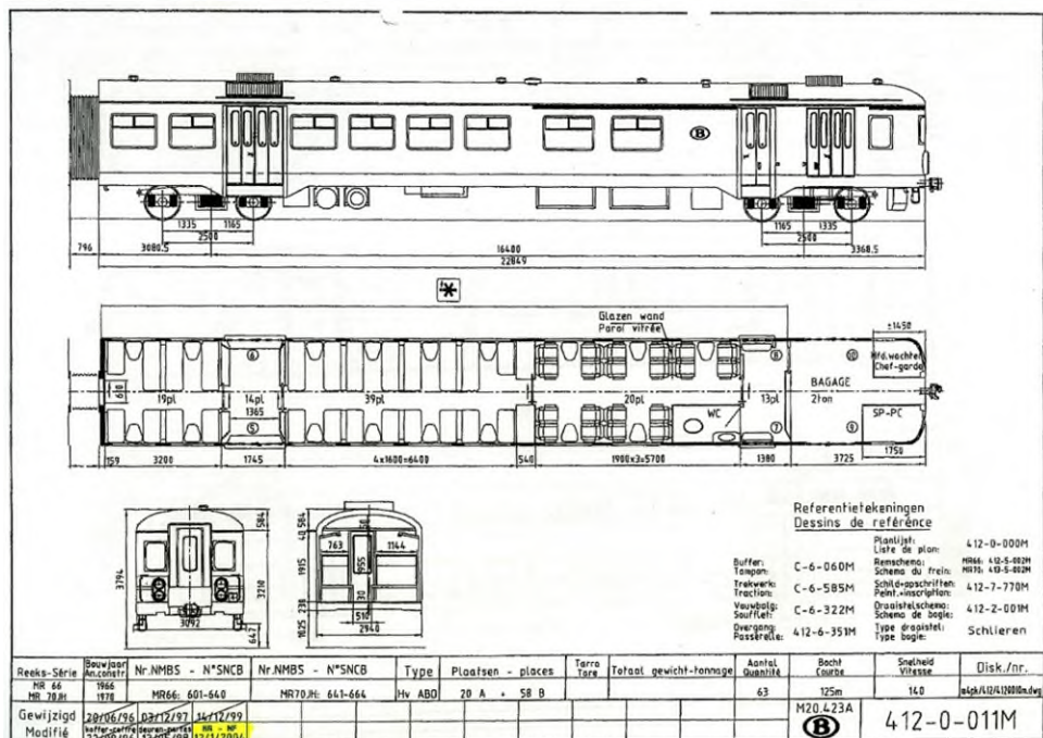
Referentietekeningen verbouwing 'New Look' 601-664 (bron: tekenbureau NMBS)
