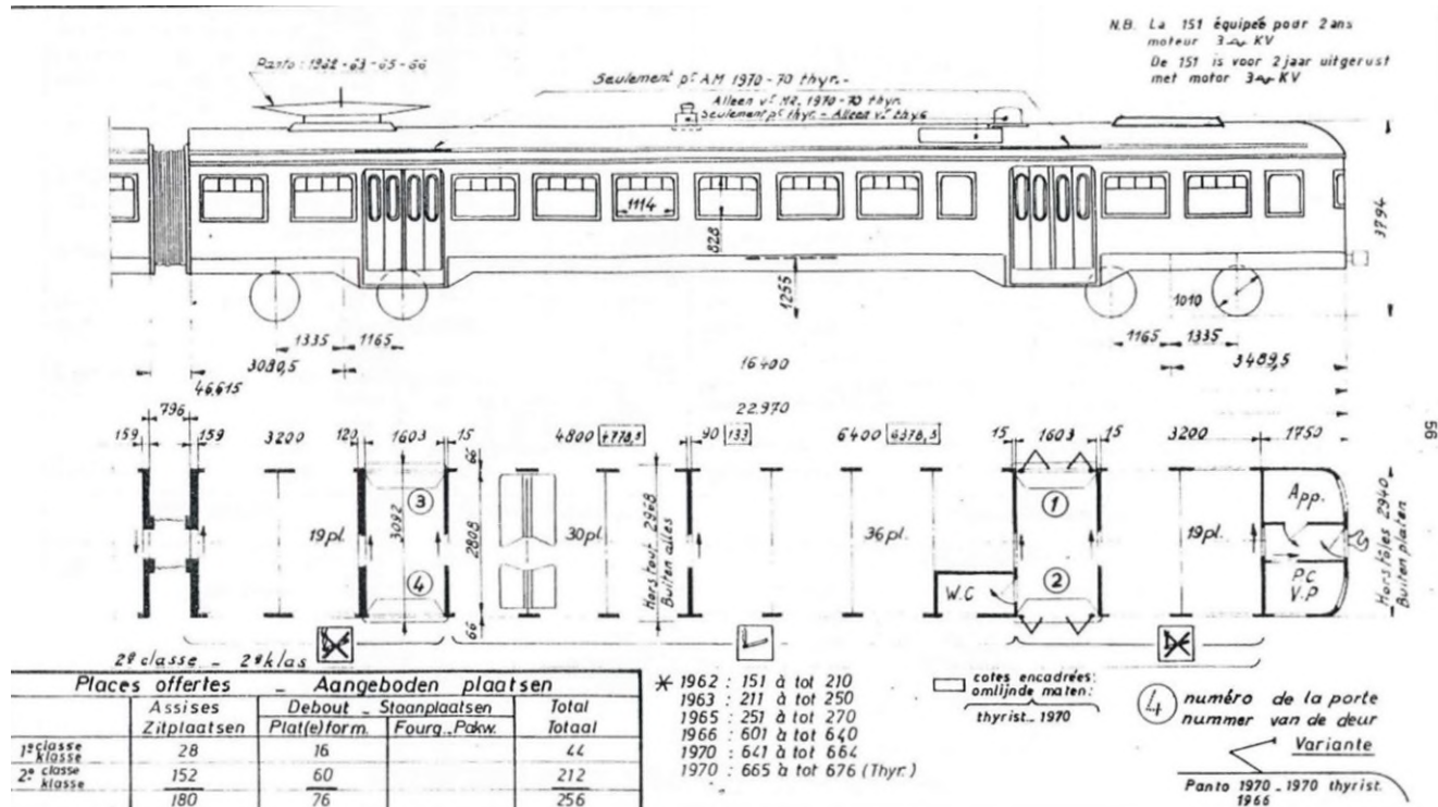
Schema van een B-rijtuig (Verzameling schema's van de motorrijtuigen van de NMBS. 1935-1986, J. Vandenberghen, 1987, p. 56.)
