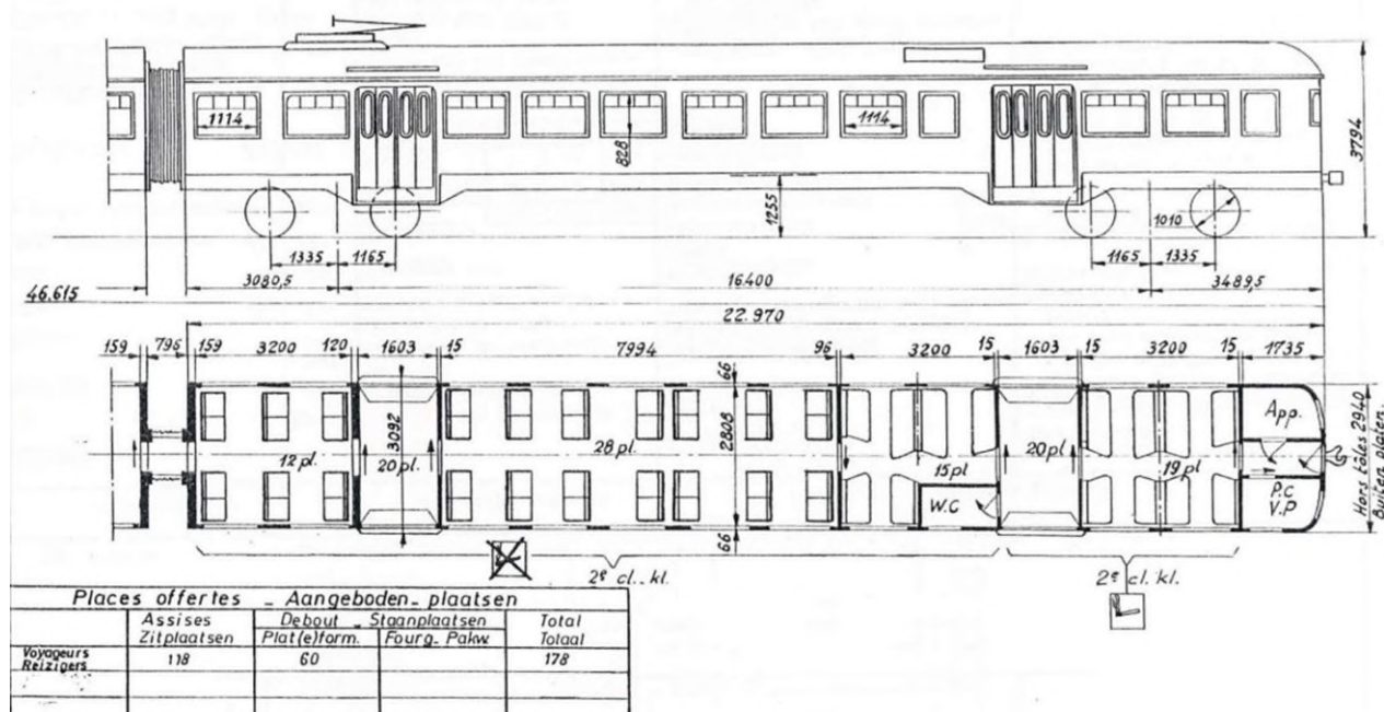
ABD-rijtuig vanaf 1979 (Verzameling schema's van de motorrijtuigen van de NMBS. 1935-1986, J. Vandenberghe, 1987, p. 62.)
