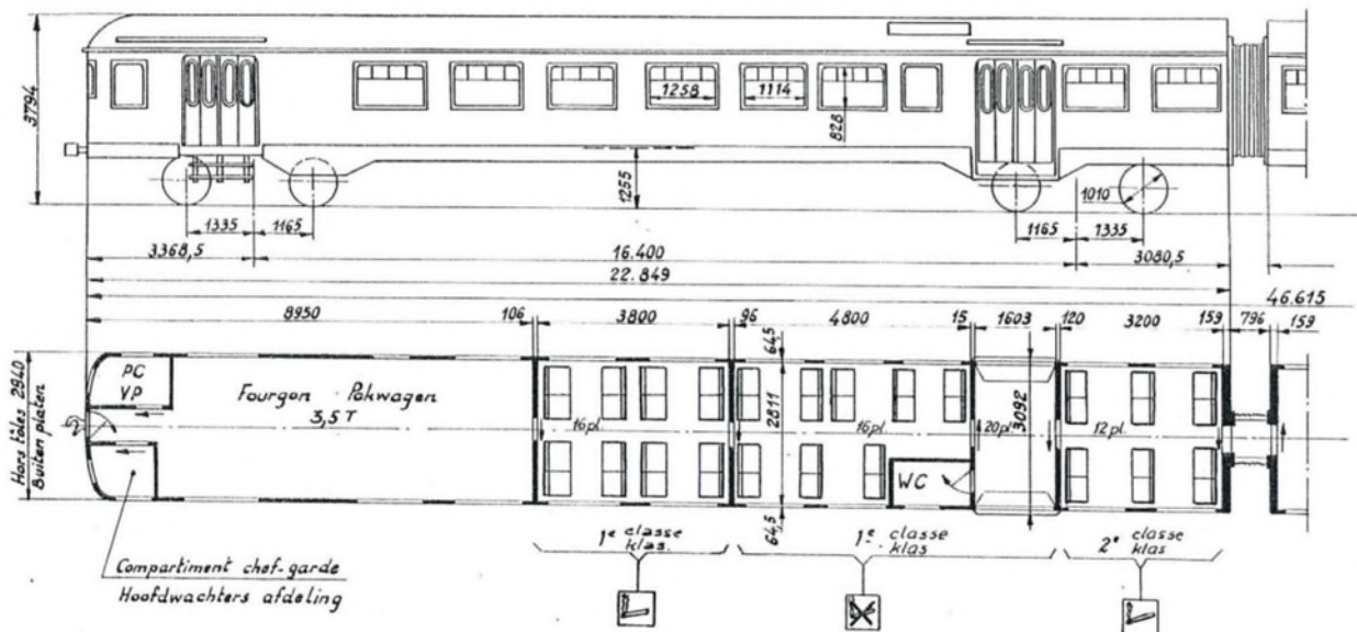
ABD-rijtuig vanaf 1979 (Verzameling schema's van de motorrijtuigen van de NMBS. 1935-1986, J. Vandenberghe, 1987, p. 62.)
