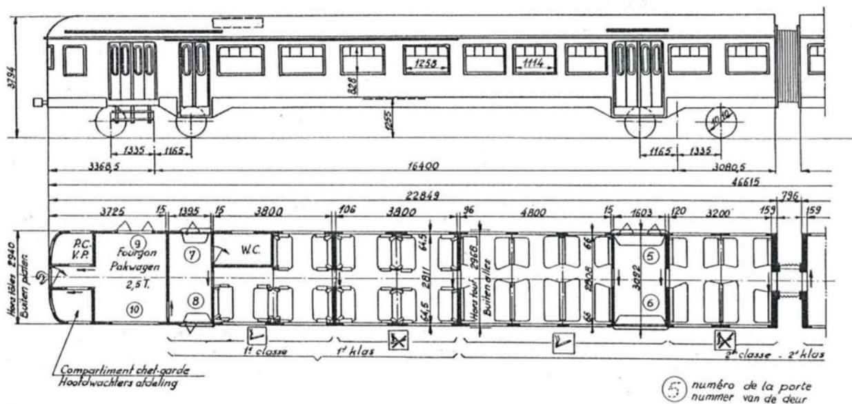
Schema van een ABD-rijtuig (Verzameling schema's van de motorrijtuigen van de NMBS. 1935-1986, J. Vandenberghe, 1987, p. 66.)
