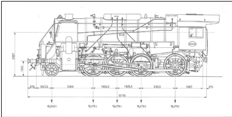
Schéma de la locomotive à vapeur type 29 « Consolidation » (Réf. I700424)
