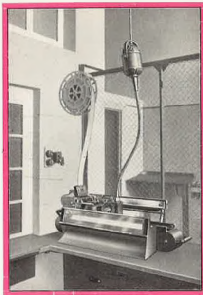
Machines à chariot mobile, type portatif, avec amenée automatique du carton et commande électrique
