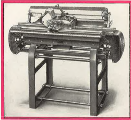
Machine à imprimer les billets à chariot mobile, Modèle G II (Notice Fd 61 sur demande)
