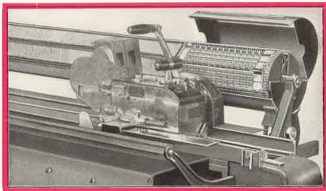
Machine à chariot mobile avec compteurs de relations
