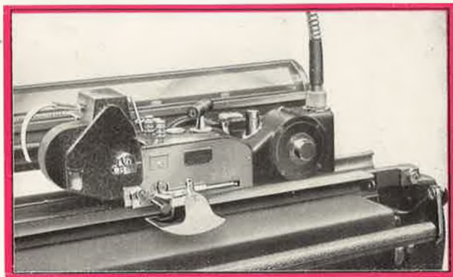
Chariot mobile, avec commande électrique
