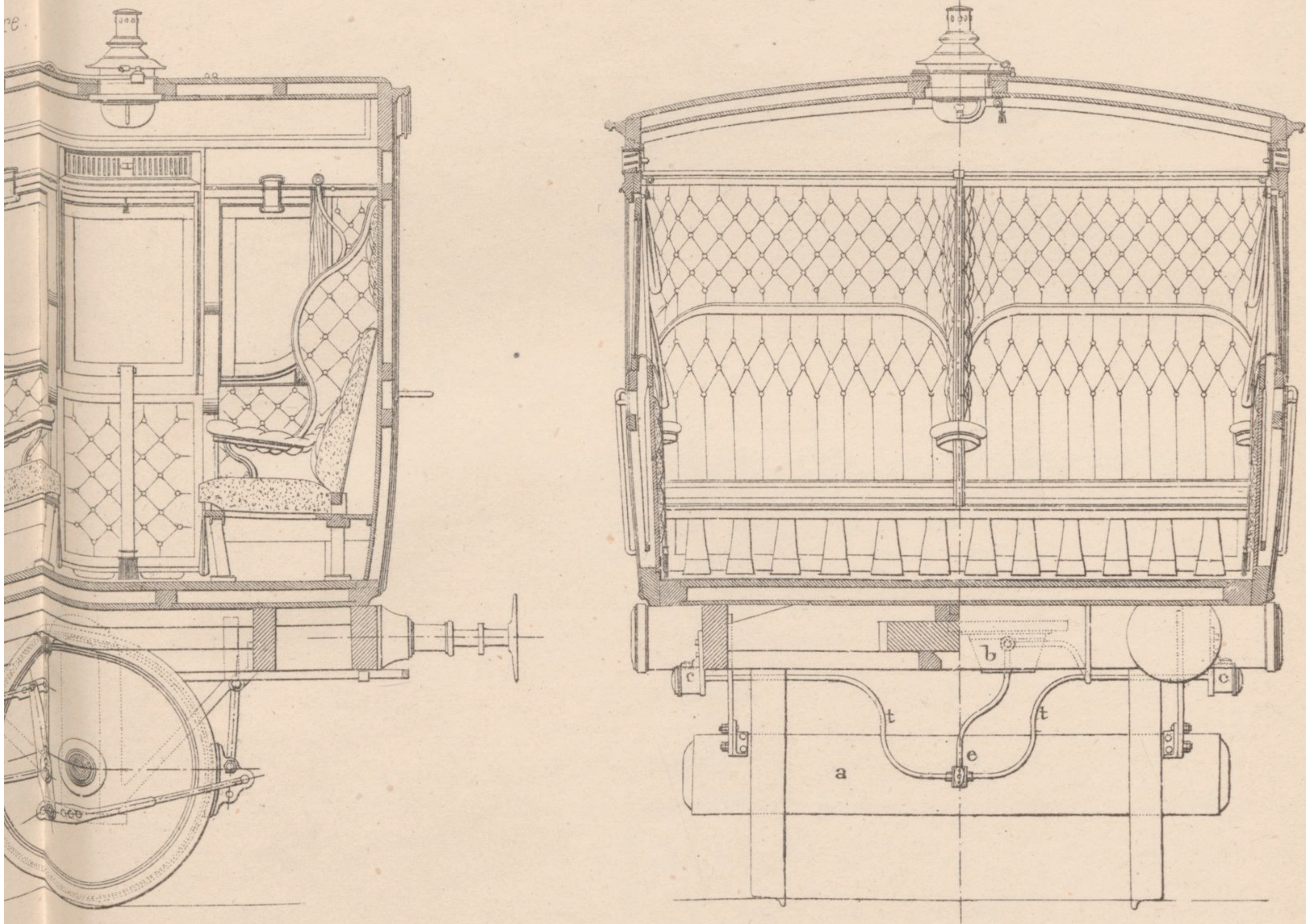
Fig. 2. Coupe transversale.
