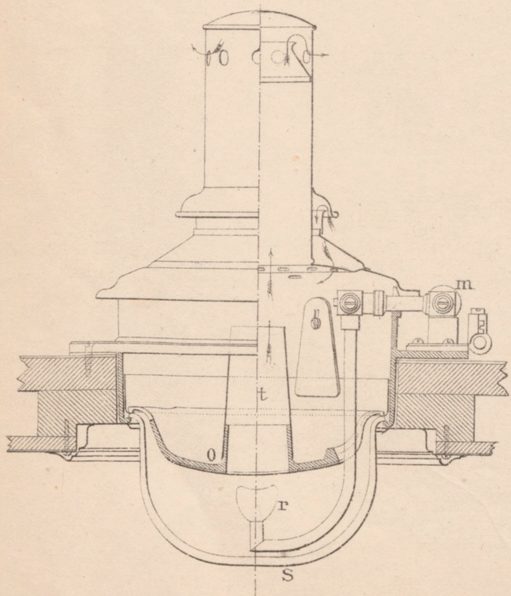
Fig.3. Lanterne de wagon.
