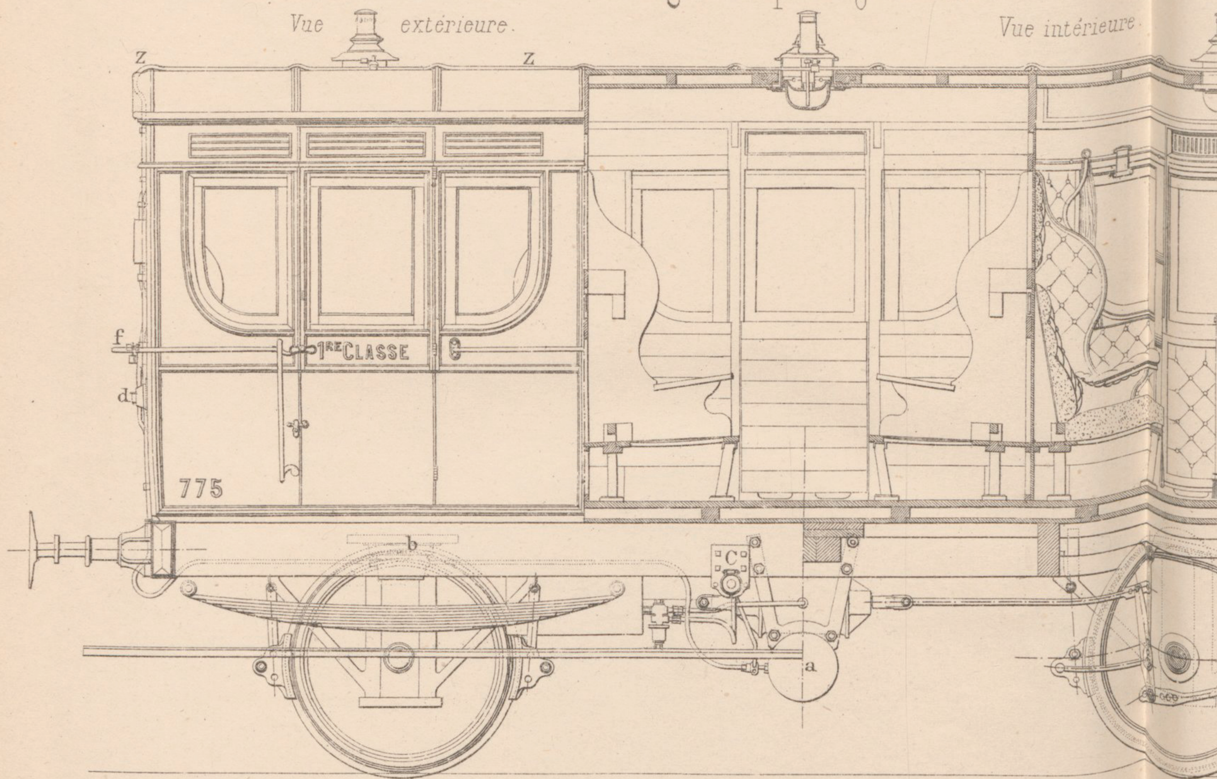
Fig.1. Coupe longitudinale.
