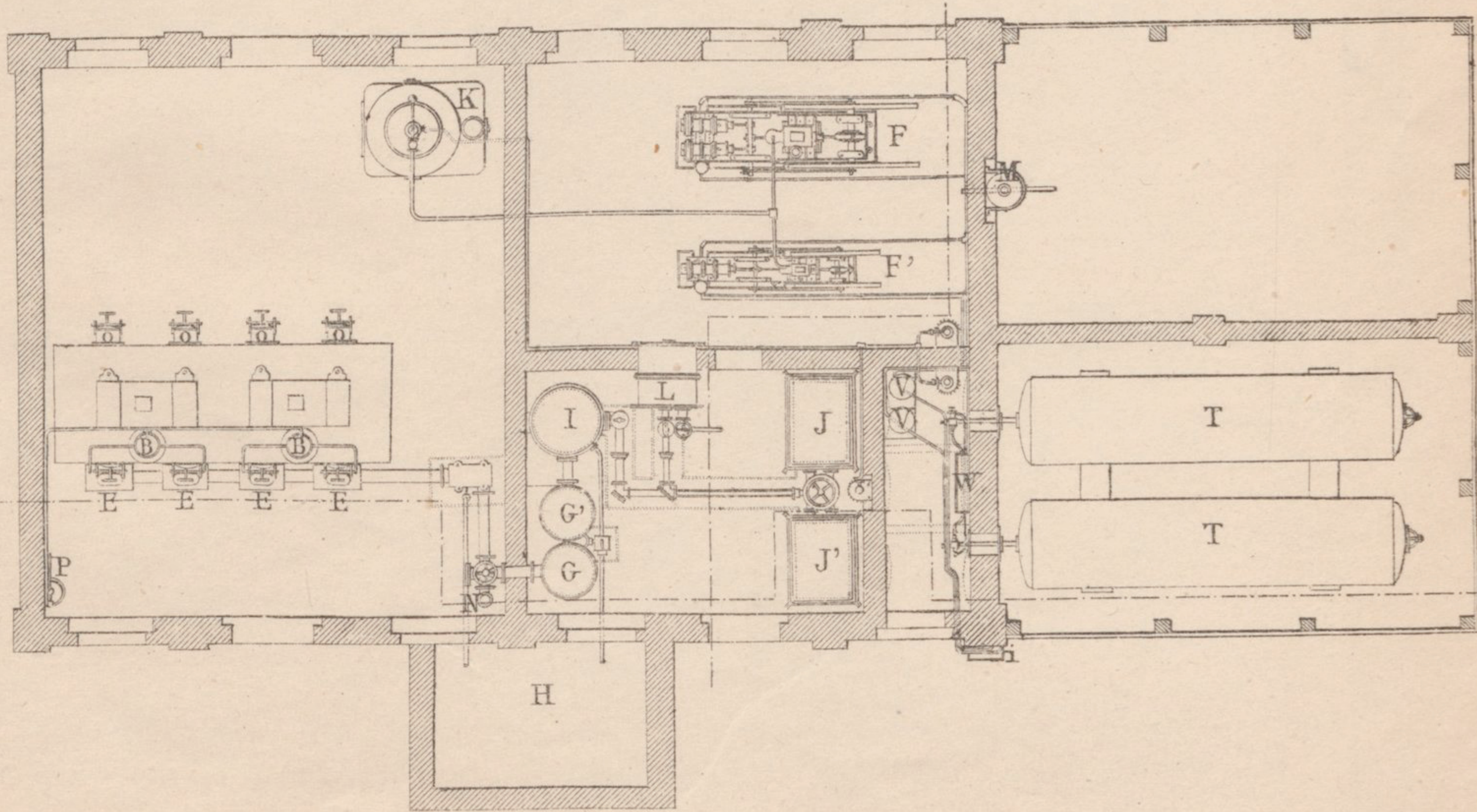
Fig. 5. Plan d'une usine à gaz .
