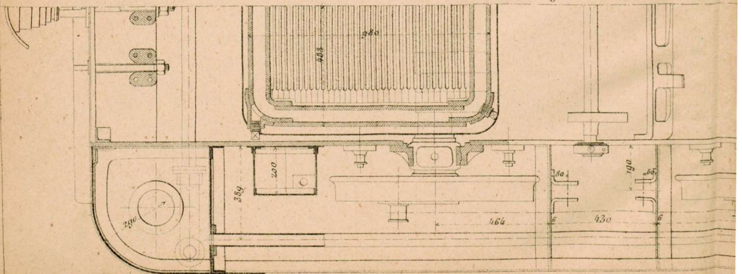
Fig.2. Demi-Plan.
