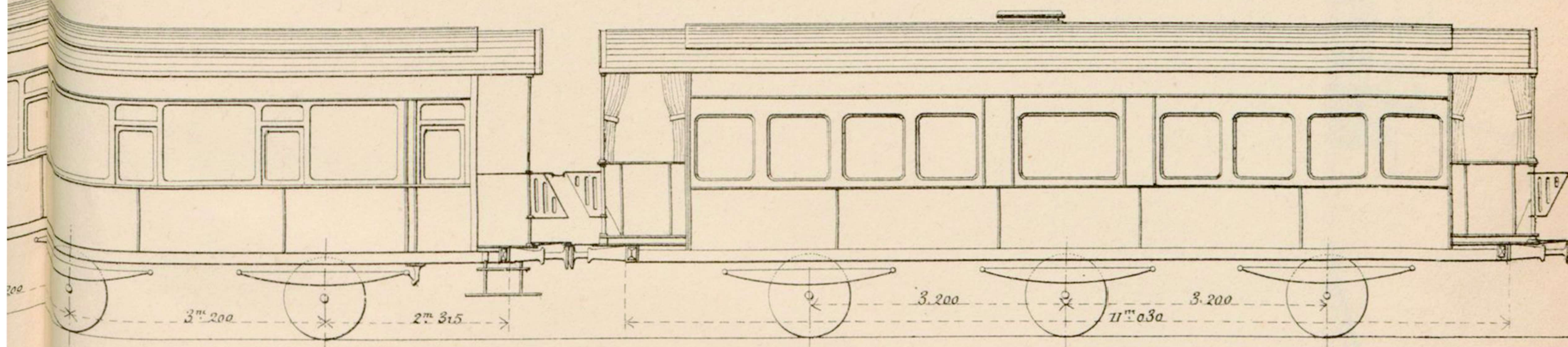
Fig. 4. Voiture-Restaurant pour 24 personnes.
