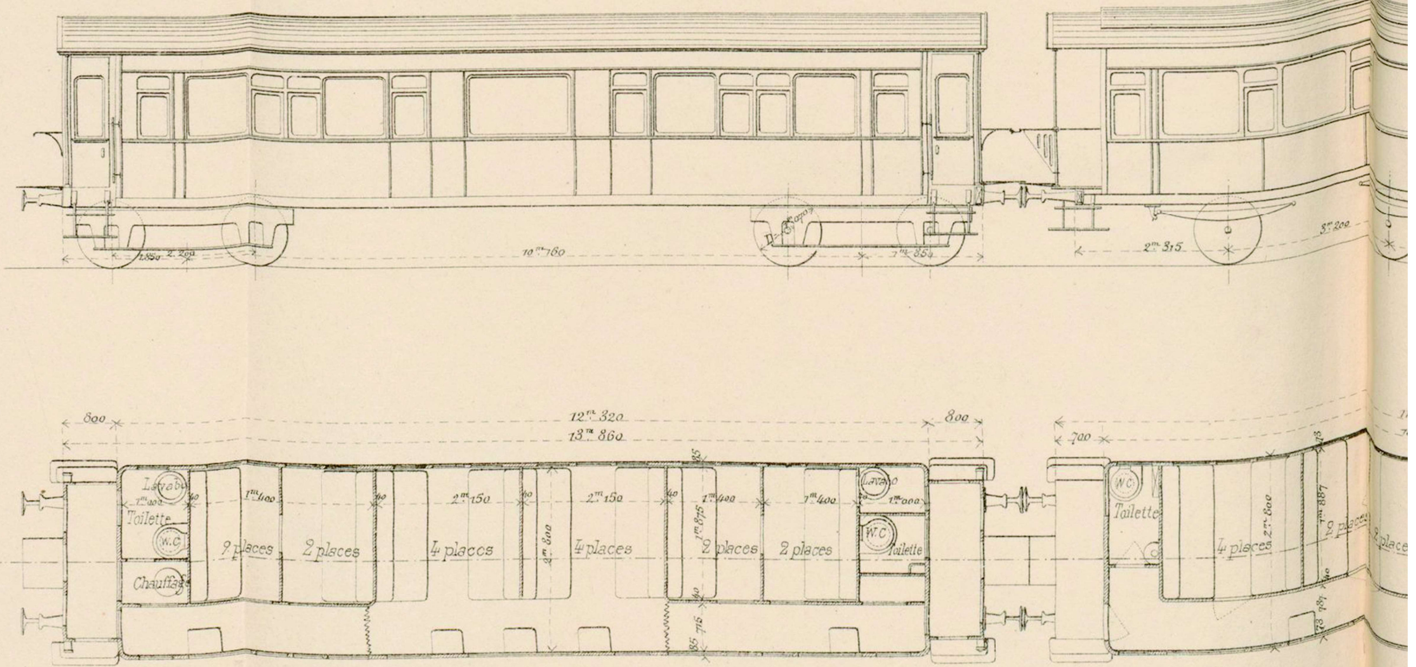
Fig.2. Voiture-Lits à 16 places, (16 Lits)
