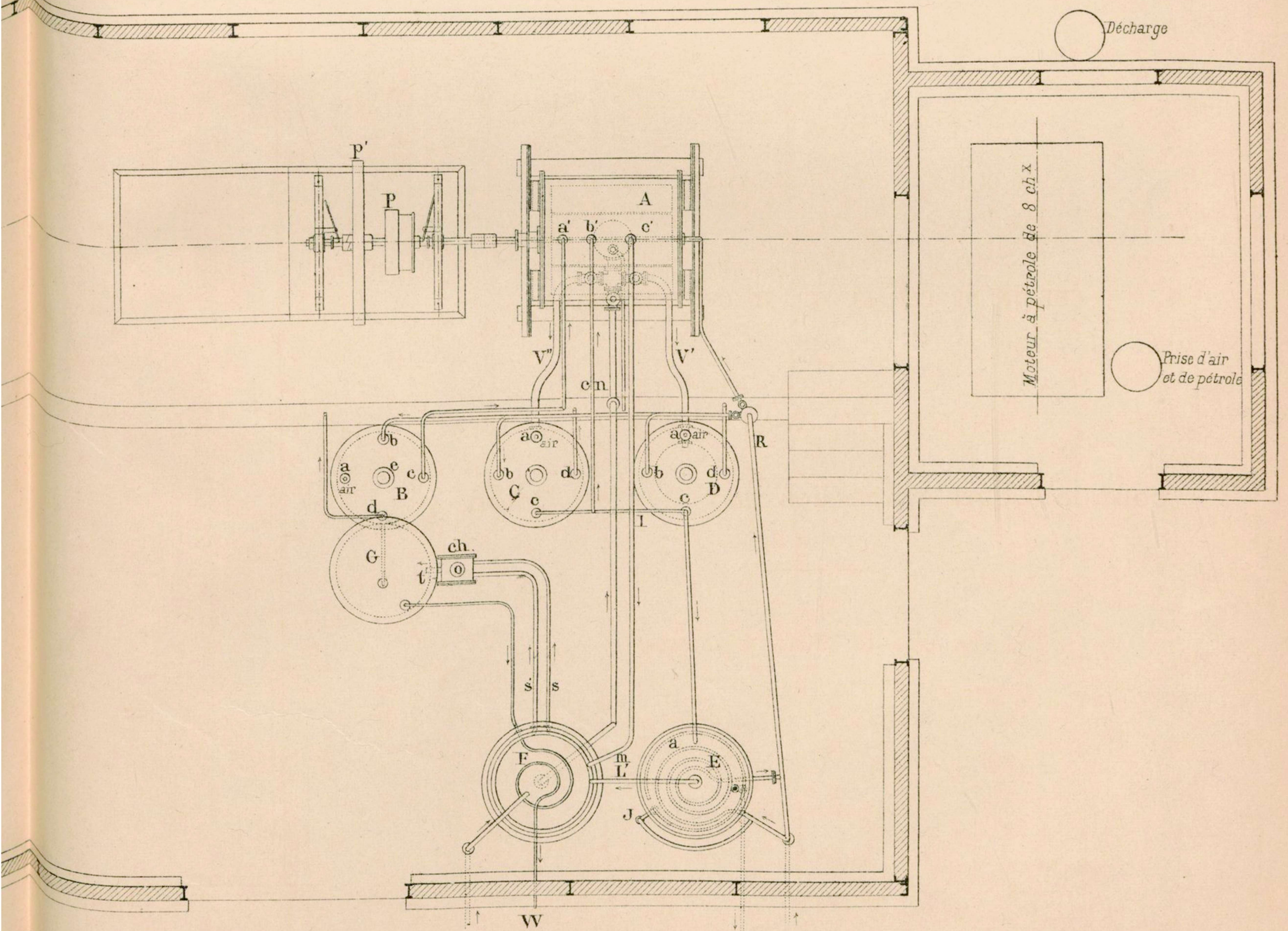
Fig. 2. — Plan
