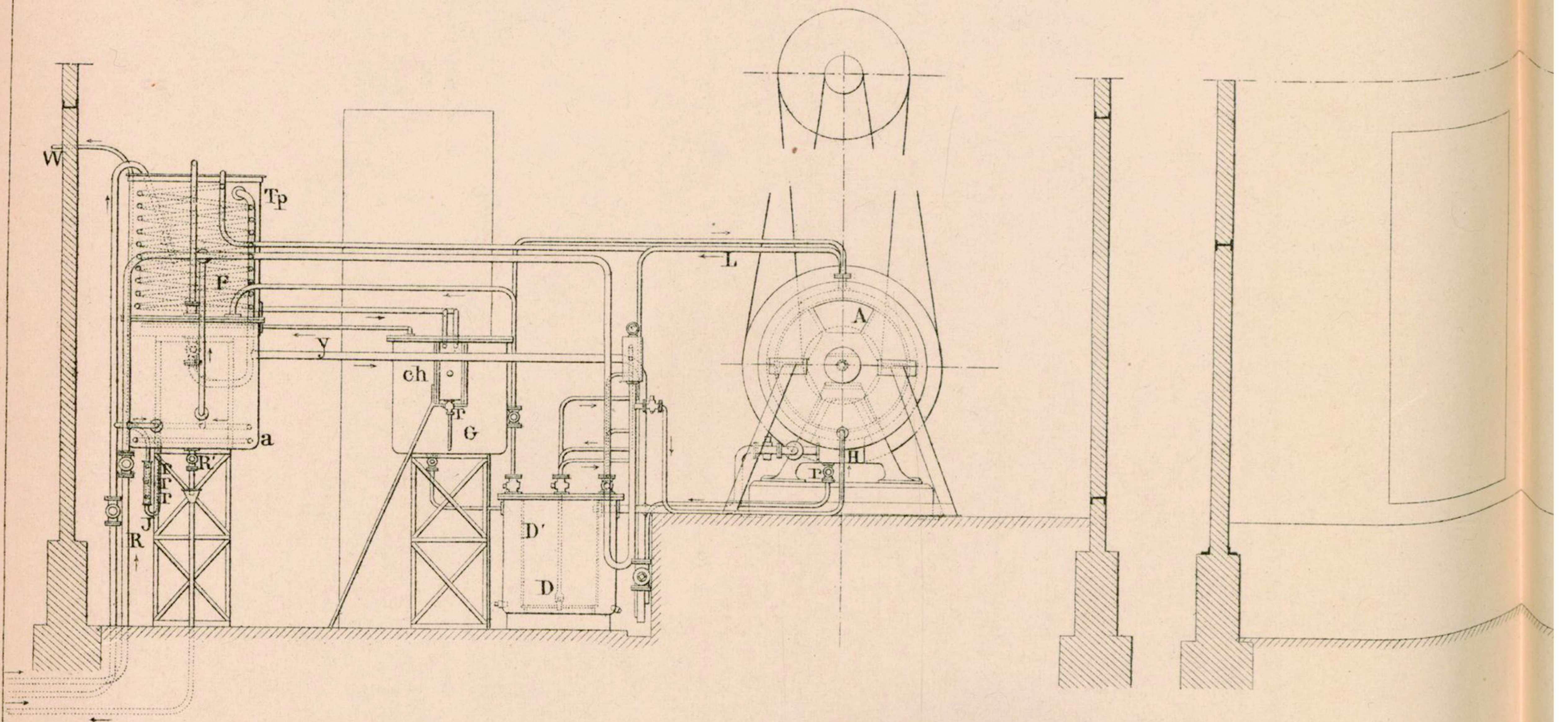
Fig. 3. — Coupe transversale.
