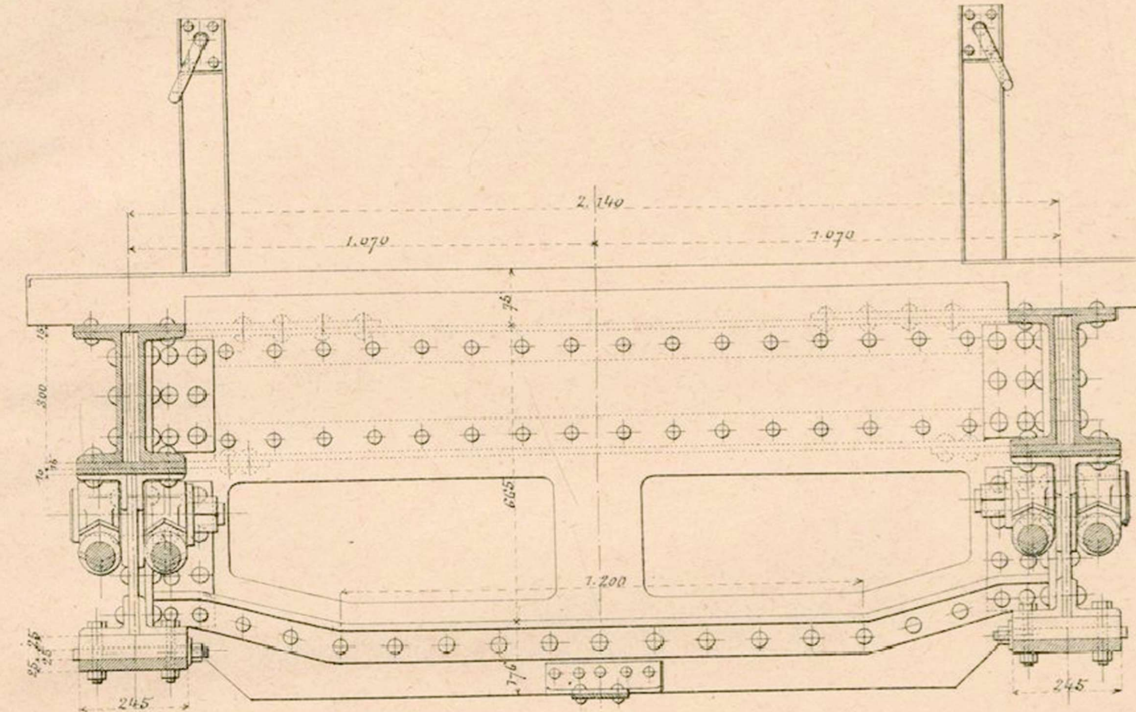
Coupe sur IJ suivant la flèche F
