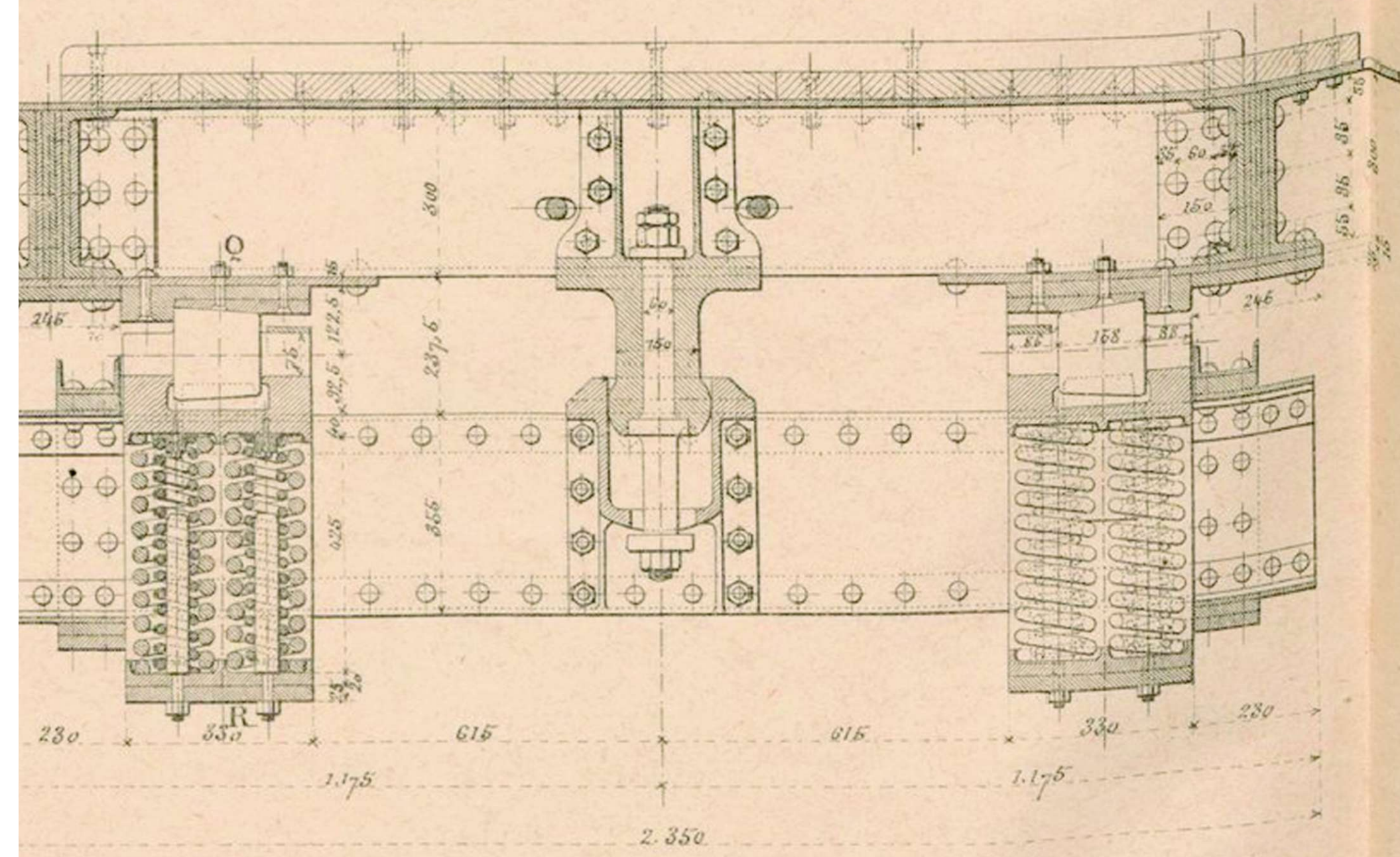
Coupe sur OP
