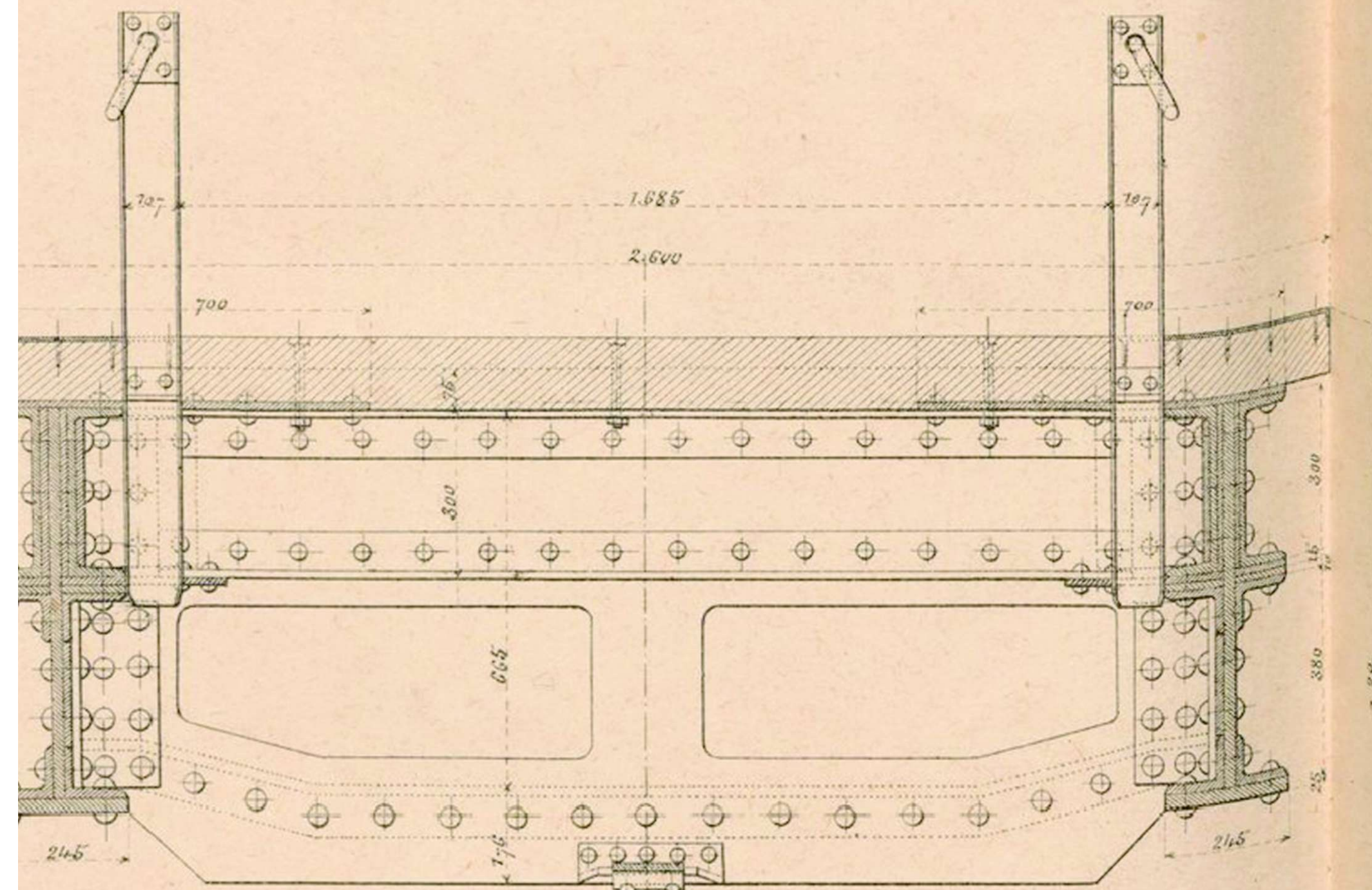
Coupe sur GH
