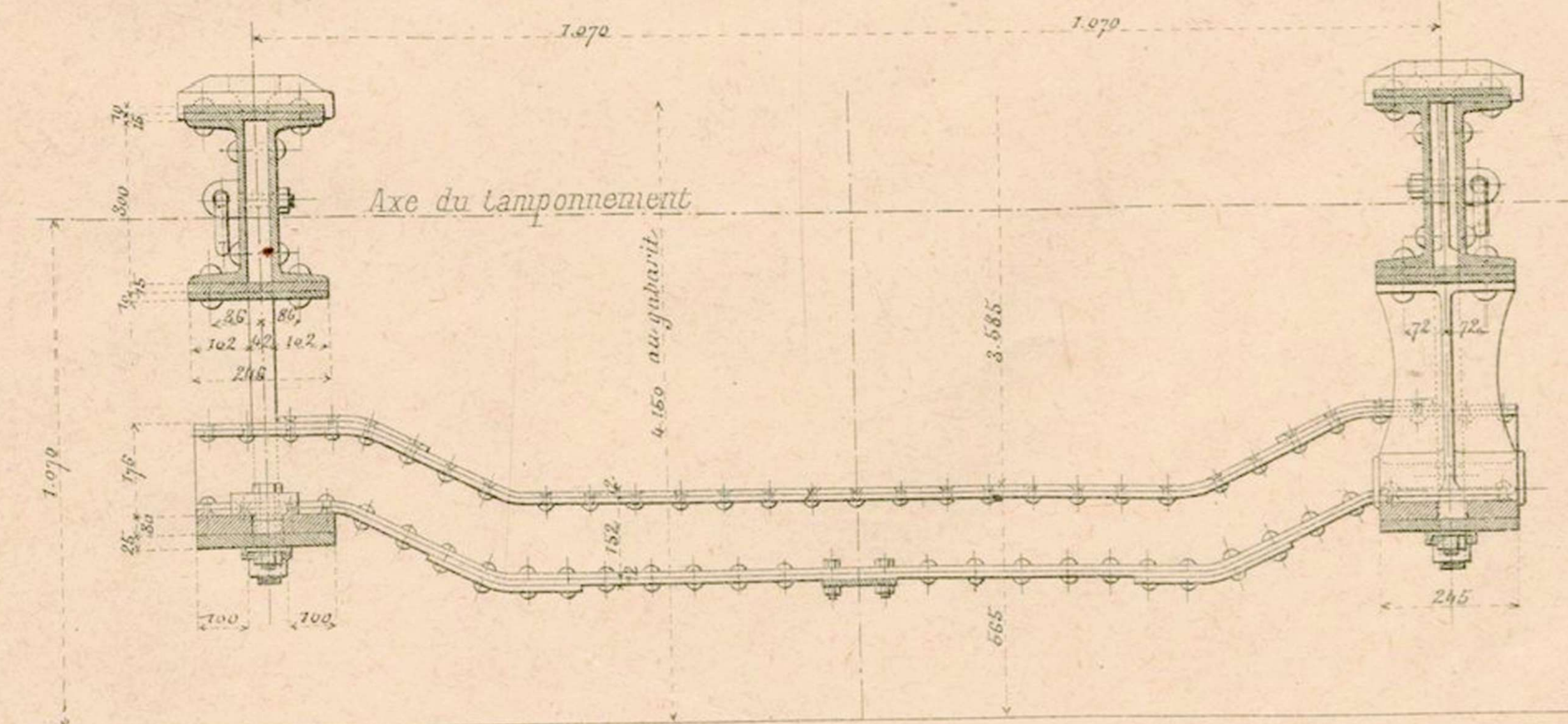
Coupe sur KLMN
