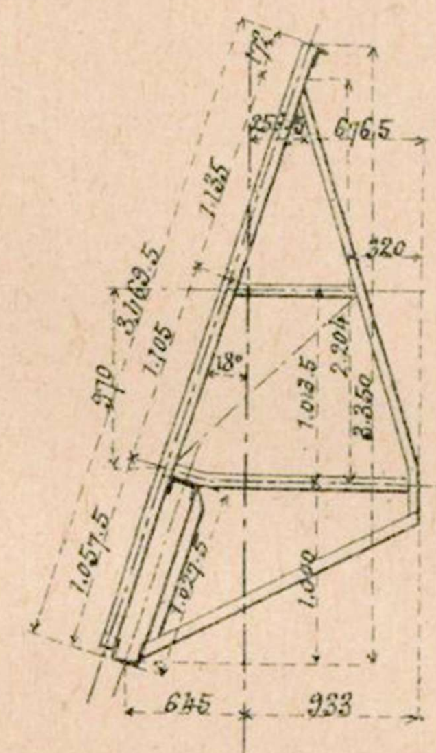
Coupe par ABCD .
