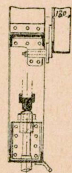
Fig. 7. Coupe suivant OP
