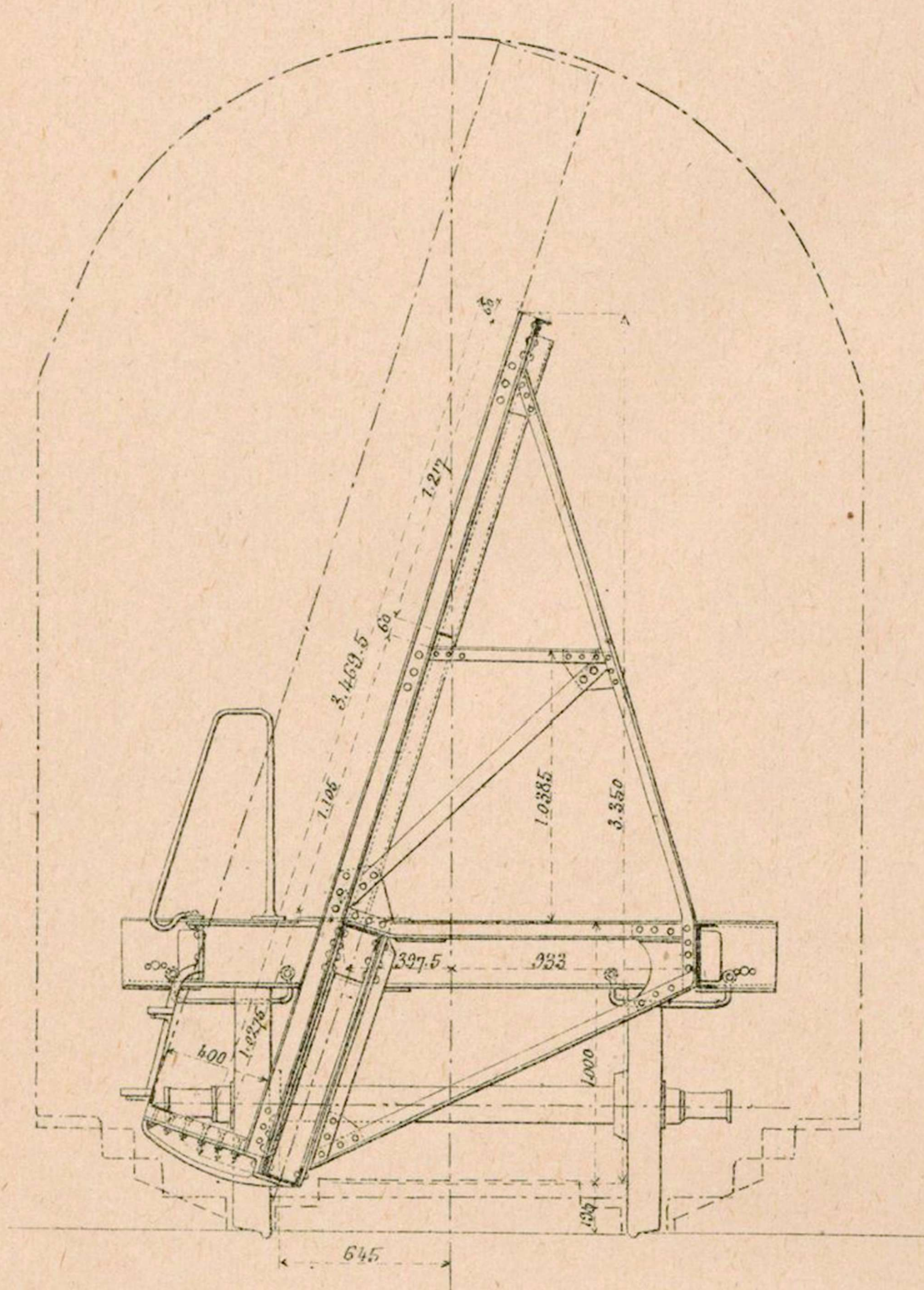
Fig. 3. Coupe transversale.
