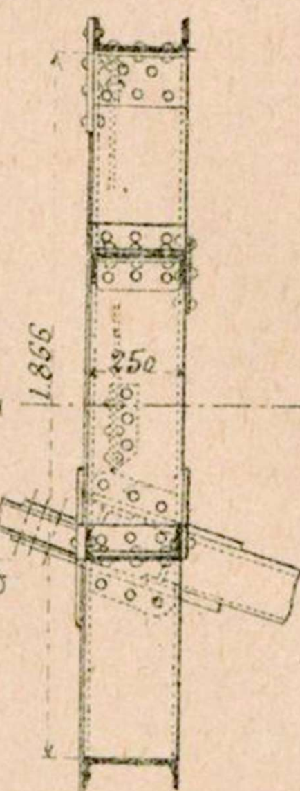
Fig. 5. Coupe suivant GH.
