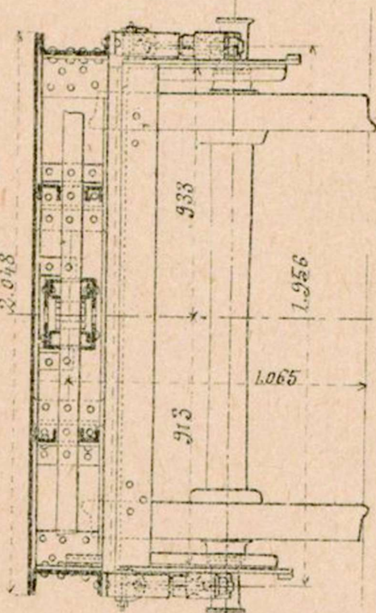
Fig. 4. Coupe suivant KLMN.
