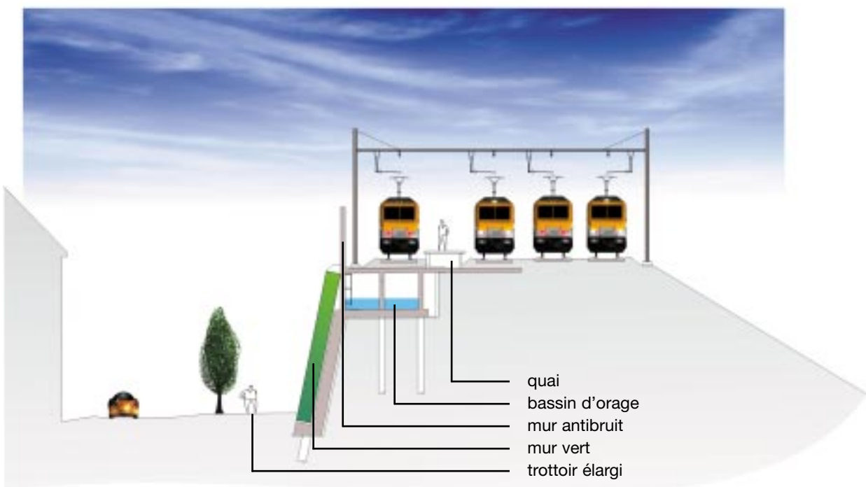
Rue des Deux Ponts: coupe de la ligne mise à quatre voies
