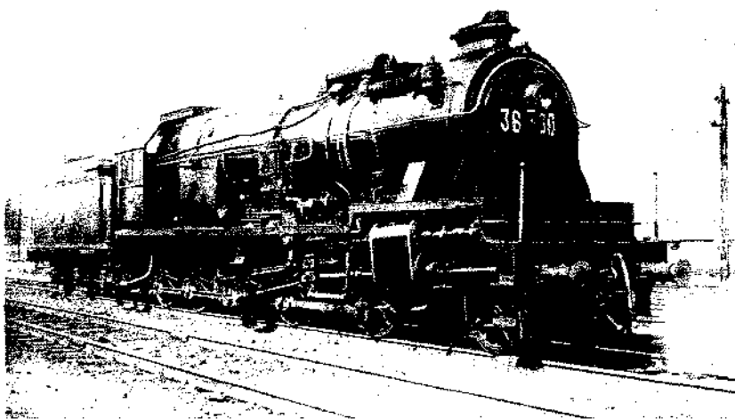
Locomotive « Decapod » type 36 - (série construite entre 1909 et 1914)
