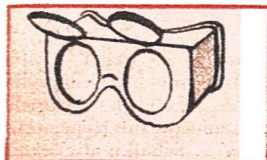
Lasbril met verstelbare gekleurde glazen en vaste heldere glazen. (Uitsnijden met automatische machine — werken met de lasbrander, snel afwisselend met het hameren).
