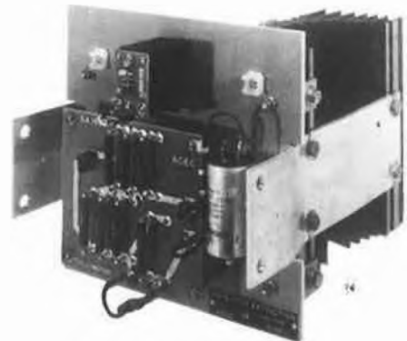
Détail d'un module Thyristor d'extinction
