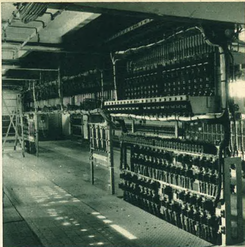
De verdieping onder het gestel van een electrisch seinhuis met wisselstraat- en seinhandels (Brussel-Zuid).
