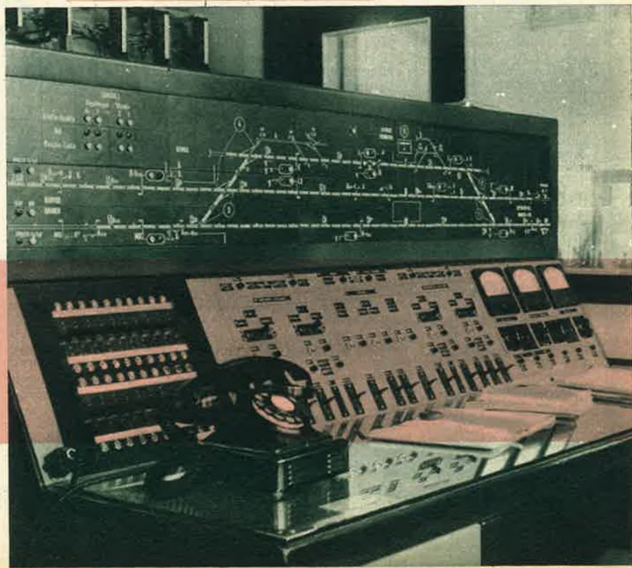
Een electrische « al-relais » bedieningspost (Terhulpen - Genval).
