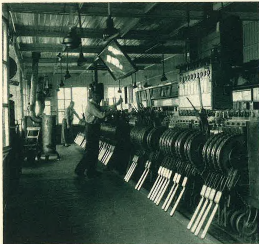
Een Siemens-seinhuis te Vorst-Zuid.
