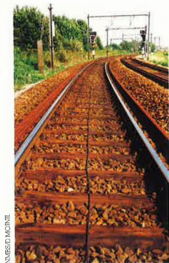
▲ KABEL WAARlangs DE SEININFORMATIE LOOPT
