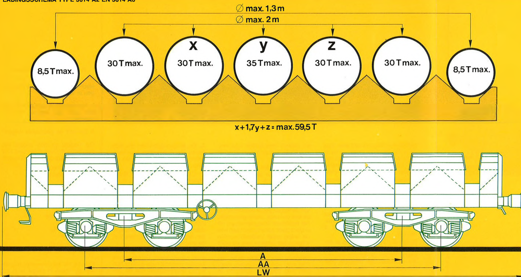
LADINGSSCHEMA TYPE 3614 A2 EN 3614 A6
