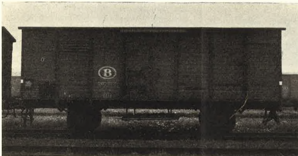
Gesloten wagon met luchtraam, 15 T.
