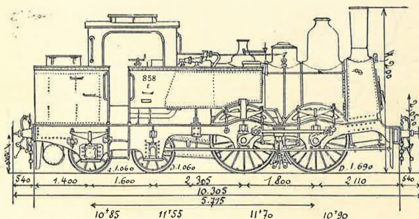
Fig. 37. — Verbouwing door de Staatsspoorwegen (n rs 856 tot 858) tot tenderlocomotieven 0-4-4-T, van de locomotieven 0-4-2 der « Grande Compagnie du Luxembourg ».
