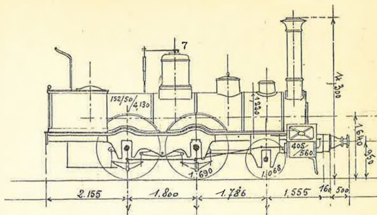
Fig. 38. — Locomotieven 2-4-0, n rs 29, 30, 31 van de « Grande Compagnie du Luxembourg », gebouwd door de « Ateliers de St-Léonard » in 1861.
