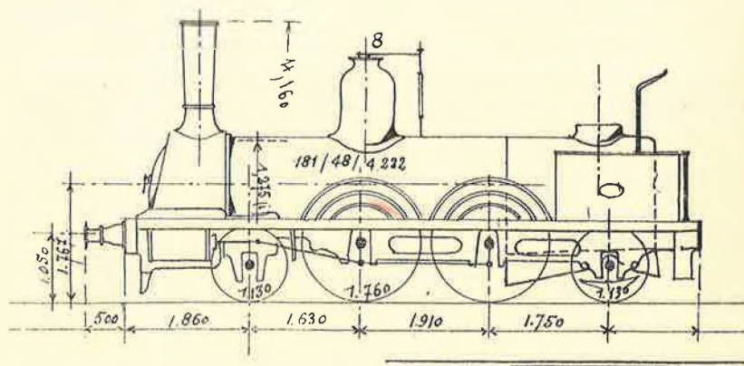
Fig. 39. — Locomotief n r 31 « La Vière », gebouwd in 1860 door R. Stephenson, van Newcastle, voor de « Grande Compagnie du Luxembourg ».
