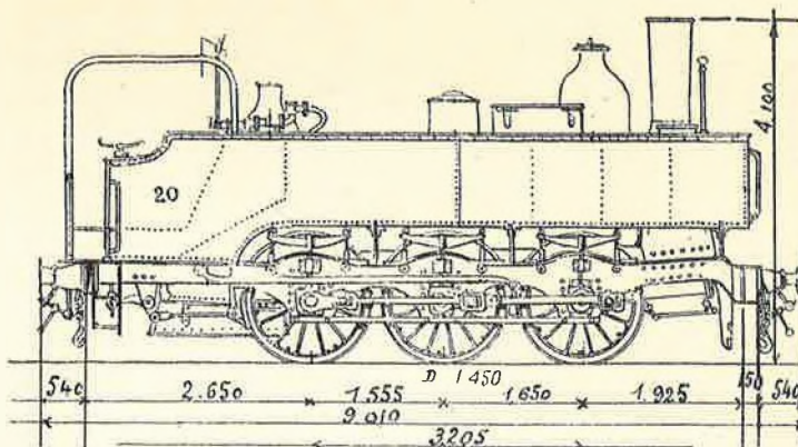
Fig. 35. — Locomotief « Belgische Staat », n° 20, afkomstig van de verbouwing tot tenderlocomotief 0-6-0-T, van de locomotief n° 9 « Ciney » met afzonderlijken tender van de « Grande Compagnie du Luxembourg », gebouwd in 1556 door de « Usines Regnier Poncelet ».
