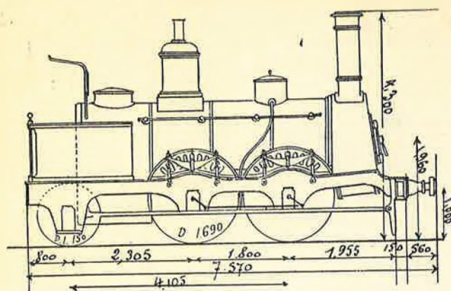
Fig. 36. — De « Recogne », de « Habay » en de « Assesse » locomotieven 0-4-2, n rs 15 tot 17 van de « Grande Compagnie du Luxembourg », gebouwd door de « Ateliers St-Léonard » in 1857.
